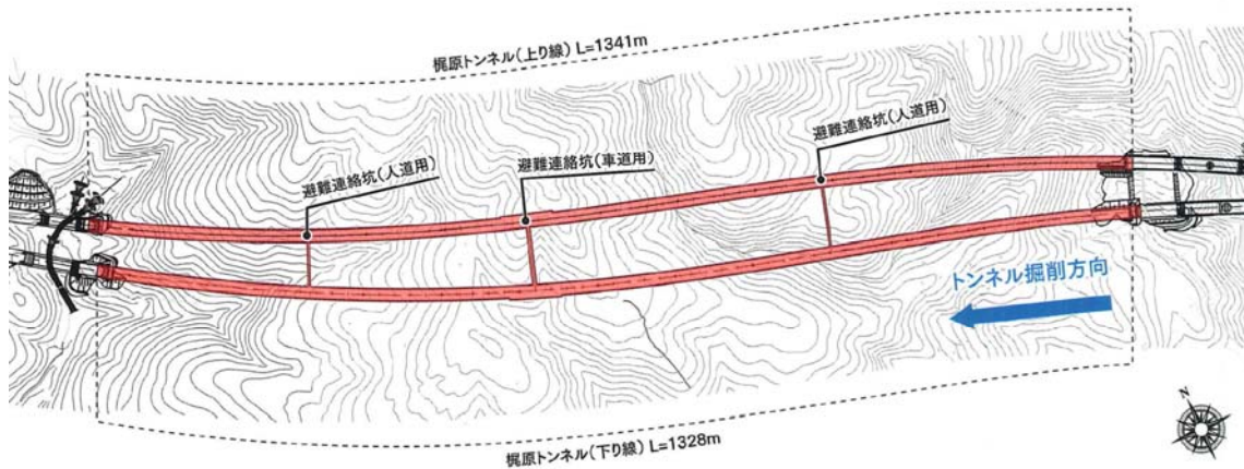
平面図
